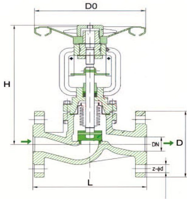
图1 波纹管密封截止阀（法兰连接）
