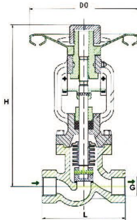
图2 波纹管密封截止阀（螺纹连接）
